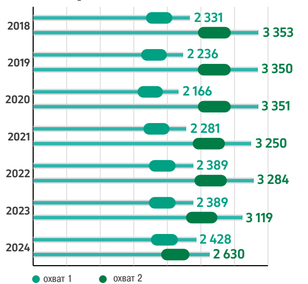
ДИНАМИКА ВЫБРОСОВ ПАРНИКОВЫХ ГАЗОВ В 2018–2024 ГОДАХ (ОБЛАСТЬ ОХВАТА 1, 2), тыс. тонн CO 2 -экв.
