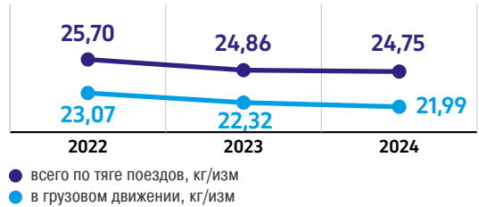
ДИНАМИКА ИЗМЕНЕНИЯ УДЕЛЬНОГО РАСХОДА ДИЗЕЛЬНОГО ТОПЛИВА НА ТЯГУ ПОЕЗДОВ, кг/изм.
